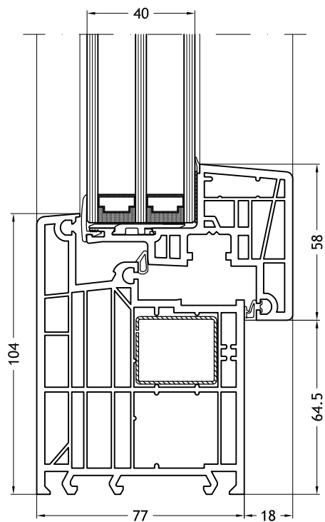
Marco Z, 964 con hoja Nova-line 953
