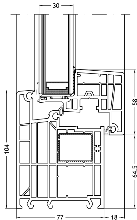
Marco Z, 964 con hoja Nova-line 971
